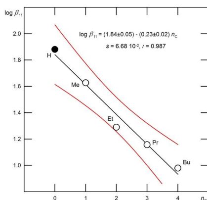
Obr. 5: Závislost logaritmu konstant stability \beta_{11} na počtu uhlíků n_C substituentu v molekule 5, Me značí methyl, Et ethyl, Pr propyl a Bu butyl, lineární regrese byla vypočtena programem OPstat, ver. 6.8 (PYTELA, Oldřich Program OPstat. Dostupné z: http://bures.upce.cz/OPgm ). Data převzata z práce: HLAVÁČKOVÁ, Kateřina. Syntéza a vlastnosti chirálních (1R,2R)-1,2-bis(1-subst.-1H-benzimidazol-2-yl)ethan-1,2-diolů. Pardubice, 2014. Diplomová práce. Univerzita Pardubice, Fakulta chemicko-technologická, Ústav organické chemie a technologie.
